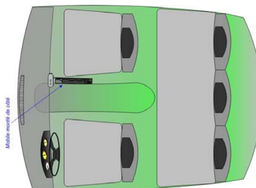
Figure 2 Représentation d'un autre montage avant avec le radio monté sur le côté de la console centrale.
