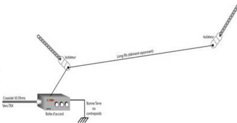
Principe d'installation d'une antenne Long Fil
